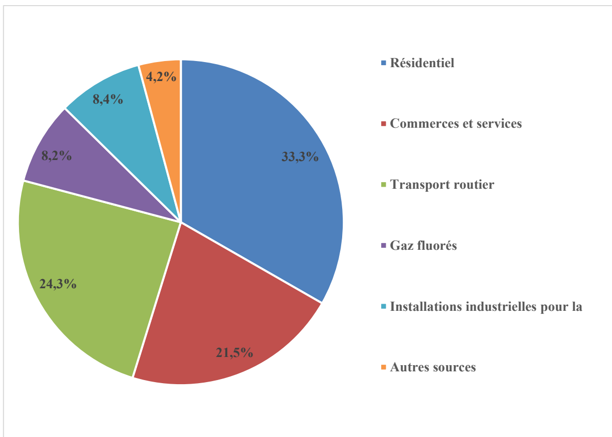
Emissions de gaz à effet de serre de la Région de Bruxelles-Capitale par secteur en 2020 (Source : Bruxelles Environnement, inventaires d'émissions 2022).
