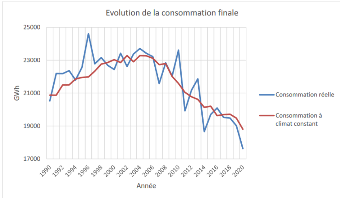
Évolution de la consommation finale totale (source : Bruxelles Environnement, Bilan énergétique régional, 2020)
